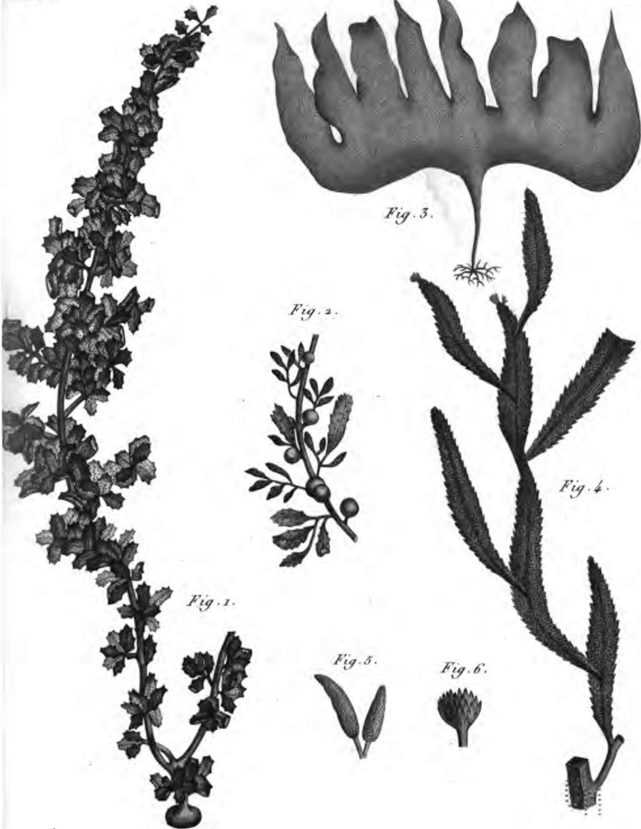
Fig. 1 Fucus foliosissimus . Fig. 2 Fucus salicifolius . Fig. 3 Laminaria reniformis Fig. 4. 5. 6 Osmundaria prolifera.
